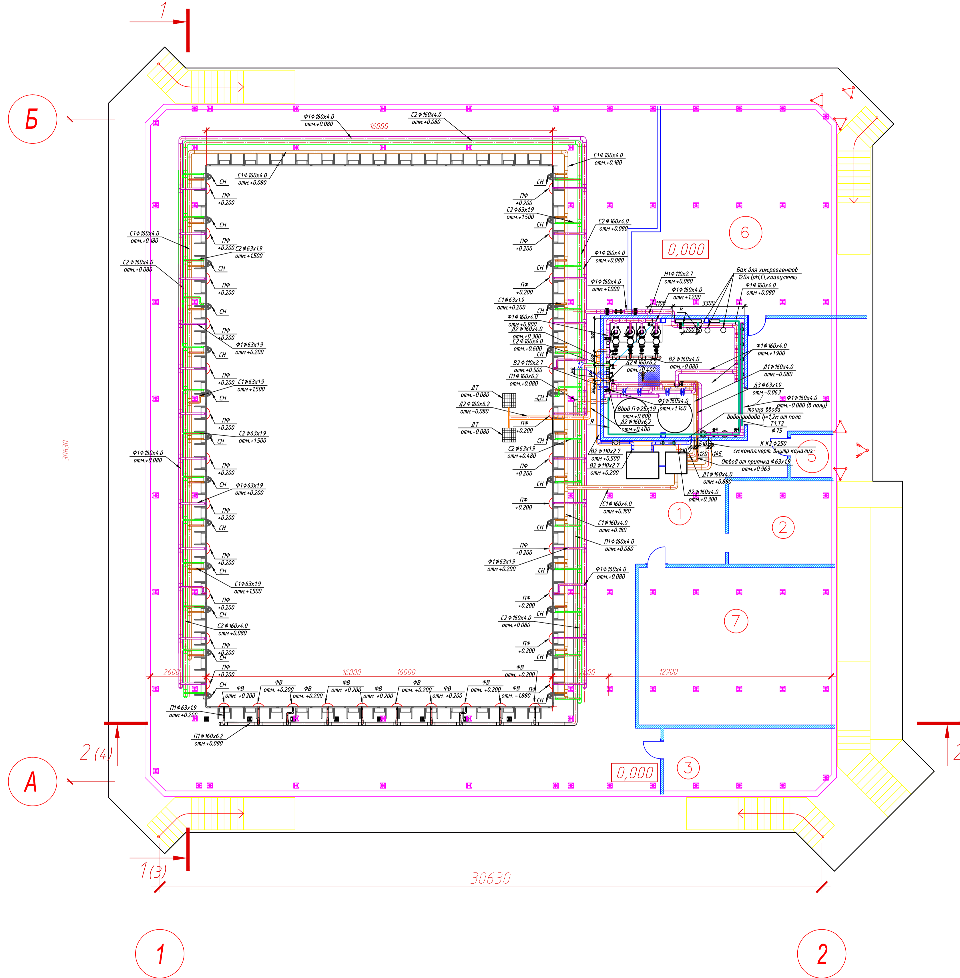
План трубопроводов на отм.0.000
